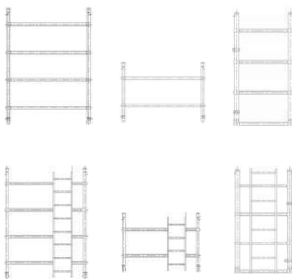
不同高度框架-双宽-2米/1.5米/1米
